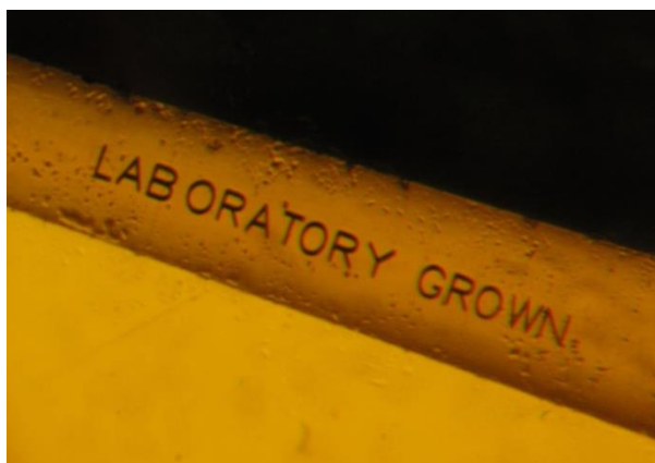
Figure 91. Inscription laser "Laboratory grown" (croissance en laboratoire) sur le rondiste d'un diamant synthétique. Photo E. Fritsch.
