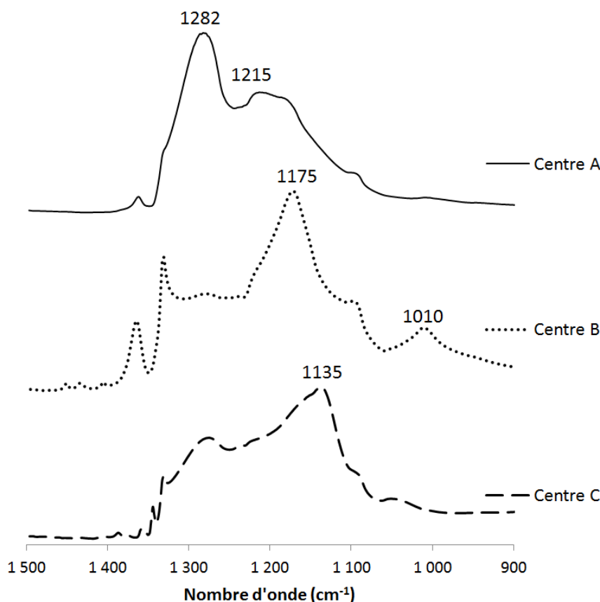
Figure 19. Spectres Infrarouge des centres A (haut), B (milieu) et C (bas). Les absorptions principales de chaque centre sont respectivement à environ 1215 et 1282 \text{cm}^{-1} , 1010 et 1175 \text{cm}^{-1} et 1135 \text{cm}^{-1} .
