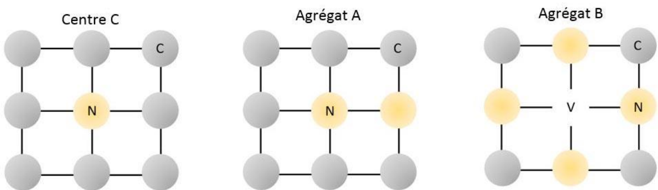
Figure 18. Schéma simplifié des défauts principaux liés à l'azote dans le diamant. En haut, le centre C correspond à un atome d'azote isolé dans la matrice du diamant. Au centre, un agrégat A, ou centre A, composé de deux atomes d'azote voisins. En bas, un agrégat B, ou centre B, correspondant à quatre atomes d'azote entourant une lacune.
