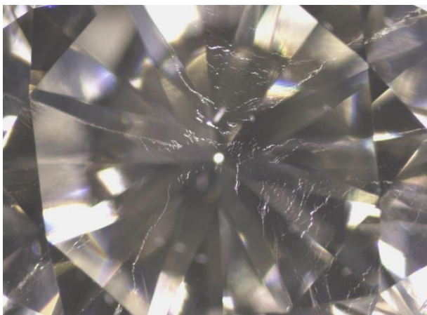
Figure 46. Twinning wisps, grossissement x20. Les twinning wisps sont définis comme des zones nuageuses produites par la distorsion du cristal, habituellement associés à des plans de déformation. Photo © Laboratoire Français de Gemmologie.
