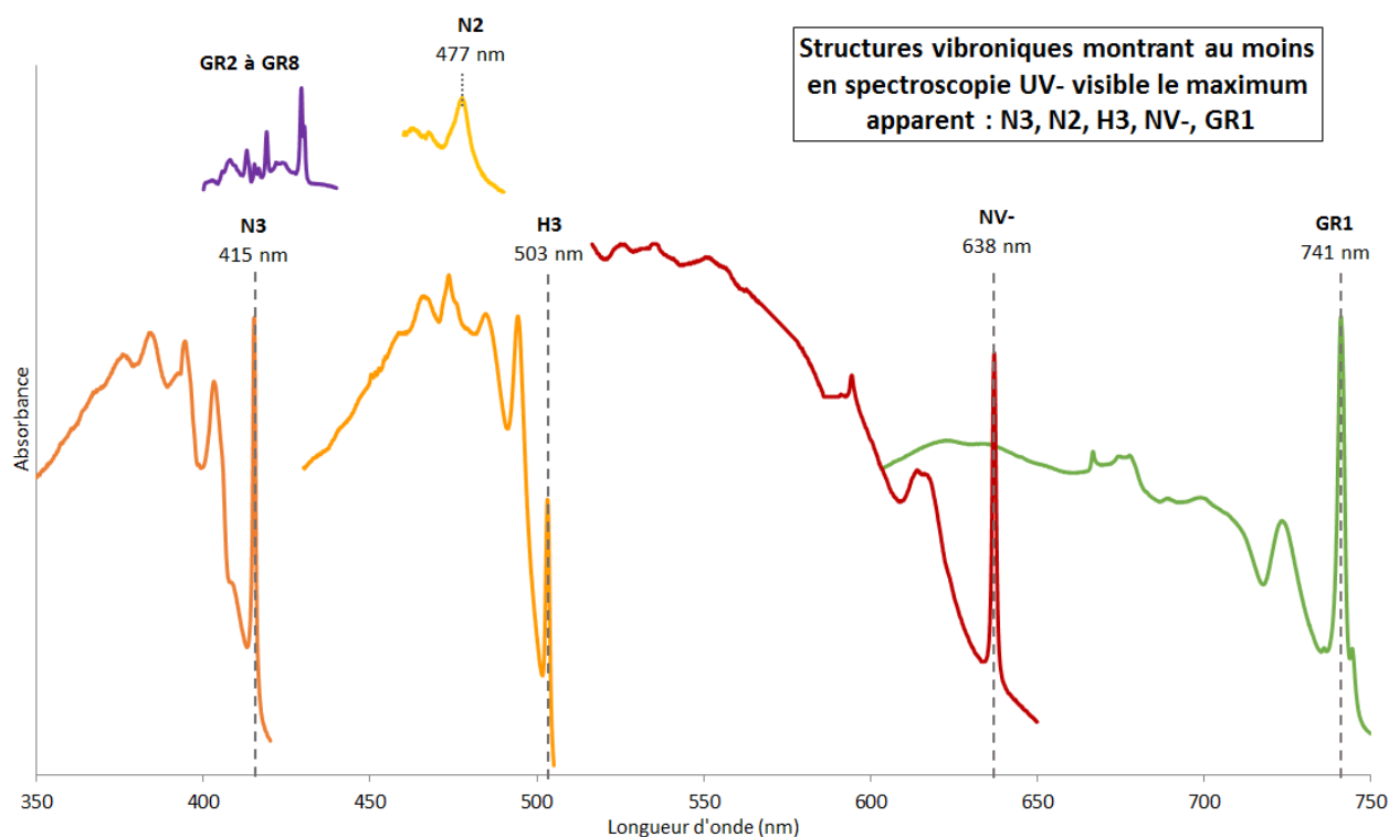
Figure 24. Principaux centres observés en spectroscopie UV-visible. La position de la ligne à zéro phonon est indexée. La majorité des centres présente des absorptions derrière cette absorption intense, nommées structure vibronique.
