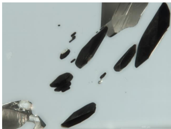
Figure 98. Inclusions métalliques orientées dans un diamant synthétique HPHT. Ces inclusions sont des restes du solvant. Elles apparaissent noires et opaques avec des formes diverses, arrondies, allongées ou irrégulières.
