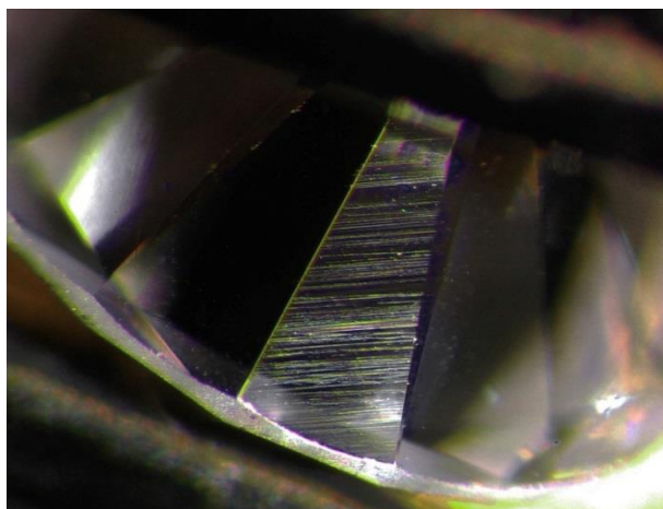
Figure 72. Stries de polissage à la surface d'un diamant. Figure 73. Marques de brûlures créées lors de l'échauffement du diamant lors du polissage. Photo F. Notari
