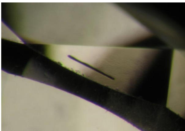
Figure 97. Inclusion typique en aiguille de métal fondu dans un diamant synthétique HPHT incolore. Photo E. Fritsch.
