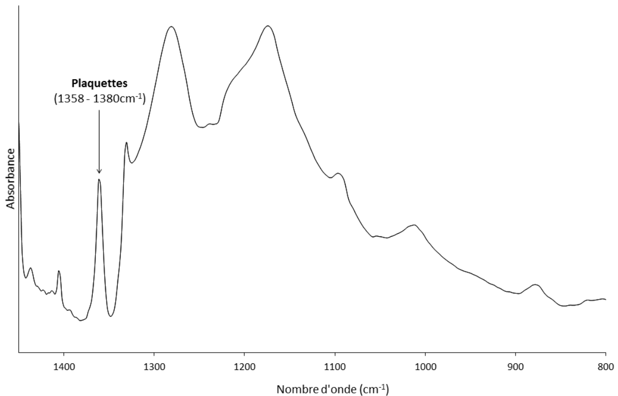
Figure 20. Spectre infrarouge d'un diamant IaAB comportant des plaquettes qui sont un défaut planaire composé de carbone et d'azote. L'absorption infrarouge de ces dernières est située entre 1358 et 1380 \text{cm}^{-1} .
