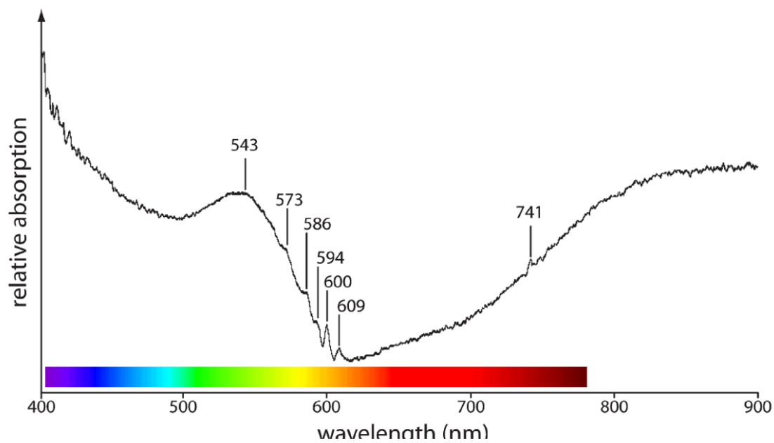
Figure 6. Spectre d'absorption dans l'UV-visible-proche infrarouge du Grand Condé. La bande large dont le maximum apparent se situe à 543 nm est responsable de la couleur rose du Grand Condé. Des pics d'absorption, situés à 573, 586, 594, 600 et 609 nm, ont été trouvés dans seulement trois diamants rose à rouge-brun. Modifié d'après Fritsch et al. (2007).
