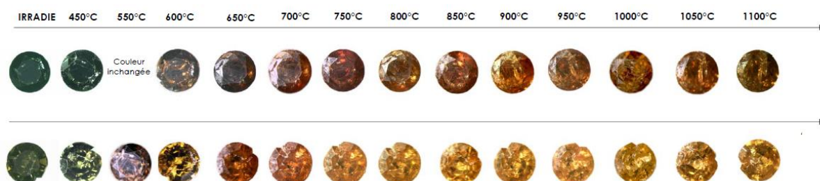
Figure 85. Évolution de la couleur de diamant précédemment irradié soumis à un chauffage. Ces diamants sont de types IaAB. La couleur passe du vert à jaune ou brun pendant le chauffage. Photo A. Respinguer. D'autres exemples sont présentés dans le mémoire de DUG d'A. Respinguer (2006).
