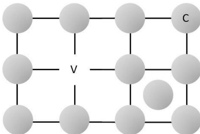
Figure 17. Schéma du centre GR1 et du centre H3. Le GR1 correspond à une lacune dans la matrice du diamant. Le centre 3H correspondant à la présence d'un atome de carbone en site interstitiel. Lors d'une irradiation des atomes de carbone se déplacent et rejoignent des intersiciels.
