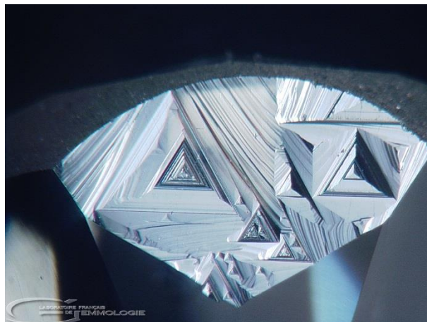
Figure 49. Trigons de dissolution à la surface d'un diamant, témoins de la forme brute, grossissement x140. Photo © Laboratoire Français de Gemmologie.
