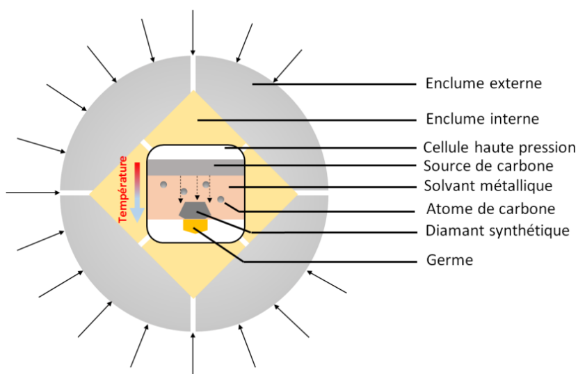
Figure 93. Schéma simplifié de la méthode Split Sphere ou "BARS". Deux enclumes entourent la cellule de haute pression au centre. La première enclume est une sphère qui forme à l'intérieur une cavité octaédrique. Dans cette cavité, une seconde enclume octaédrique forme en son centre une cavité cubique dans laquelle se trouve la cellule. Ainsi la pression créée par les enclumes est dirigée dans toutes les directions de l'espace (isotrope). De la même manière que pour la méthode "belt", un gradient de température est créé dans la cellule, permettant de cristalliser un diamant synthétique monocristallin en continuité
