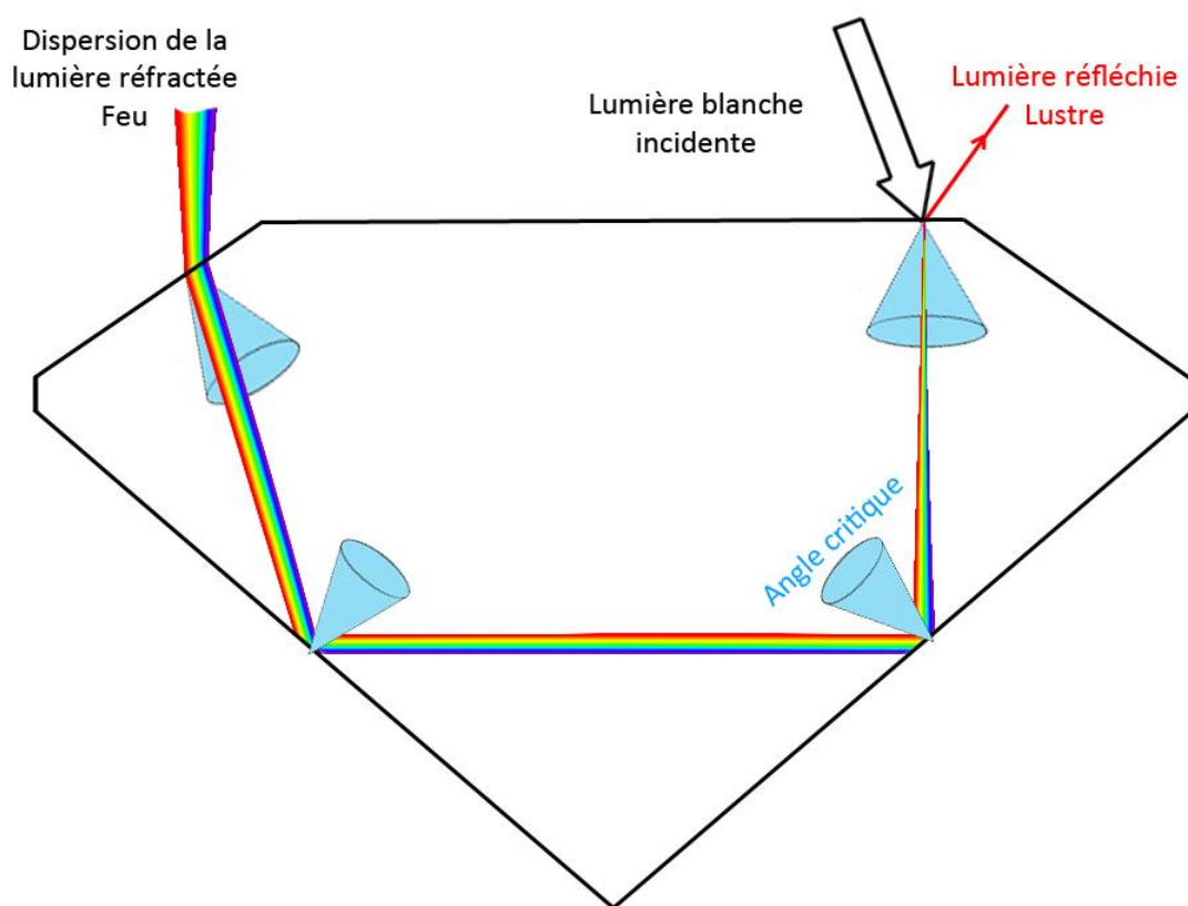
Figure 10. Schéma du chemin de la lumière dans un diamant taillé. Un rayon de lumière blanche arrivant en surface d'un diamant sera en partie réfléchi. Cette proportion de lumière va créer ce qui se nomme le lustre. La seconde partie est réfractée dans la pierre. L'enjeu est de faire ressortir un maximum de lumière vers l'œil. En traversant la pierre, les rayons lumineux sont dispersés pour créer alors les feux du diamant. L'angle critique est l'angle dans lequel un rayon lumineux peut entrer ou sortir de la pierre.
