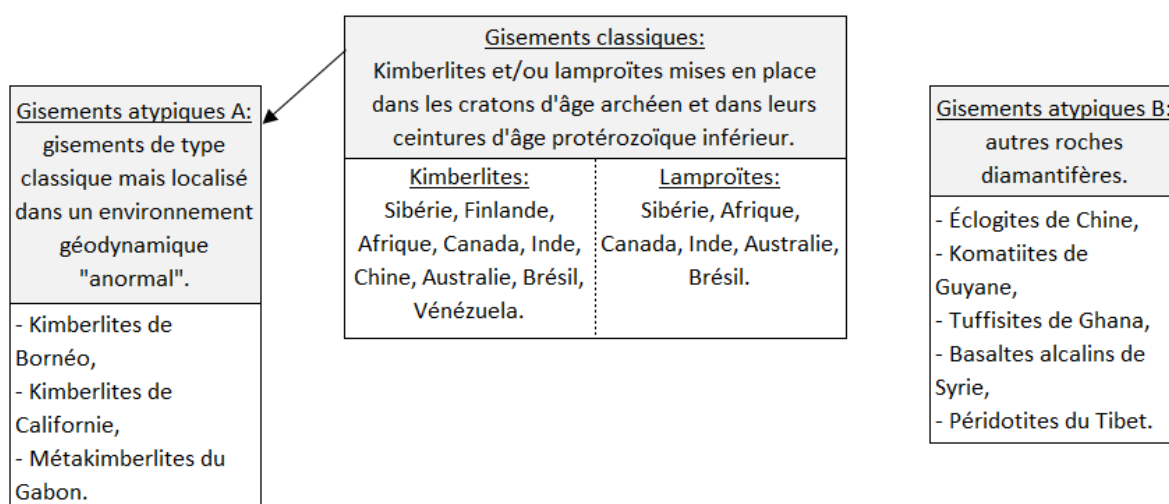
Figure 57. Typologie simplifiée des gisements primaires, modifié d'après Barthélémy et al. (2008).
