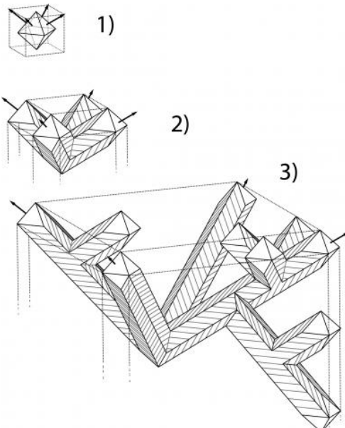
Figure 14. Schéma de la formation des fibres dans un diamant fibreux. Les fibres correspondent à des octaèdres allongés qui se ramifient jusqu'à former un cube. Schéma B. Rondeau
