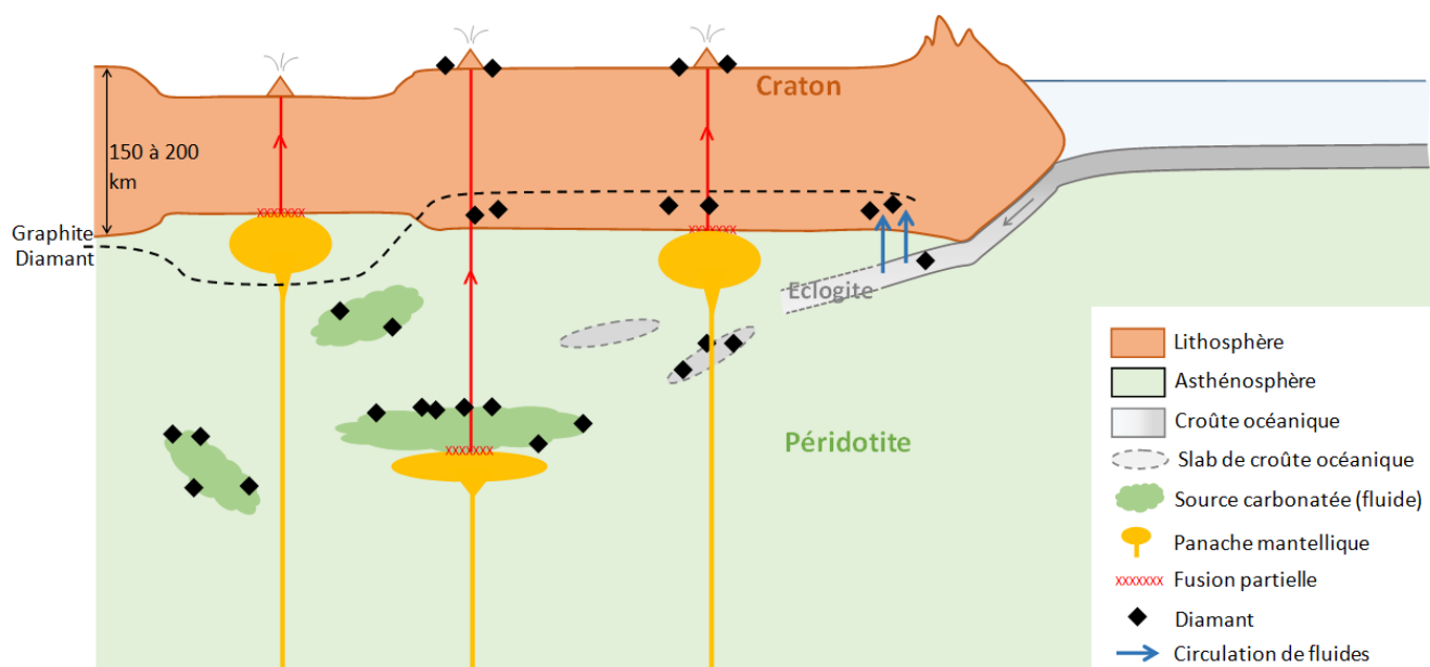
Figure 56. Schéma de la formation et du transport des diamants jusqu'en surface. Dans un premier temps les diamants se forment à la base du manteau lithosphérique et dans le manteau asthénosphérique, grâce à la présence de fluides déjà présents dans le manteau ou apportés par la croûte océanique. Leur cristallisation est possible uniquement dans la zone de stabilité du diamant (en dessous de la ligne en pointillés noirs). Les plumes, remontées ponctuelles de roches anormalement chaudes permettent la fusion partielle à la base de la lithosphère ou possiblement au contact d'une zone carbonatée générant alors la remontée d'un magma. Si ce dernier croise une zone diamantifère dans le manteau durant sa remontée alors les diamants seront apportés à la surface. Si le magma est généré sous une lithosphère plus fine (le cas le plus fréquent, à gauche) alors la kimberlite ne peut pas remonter de diamant en surface.
