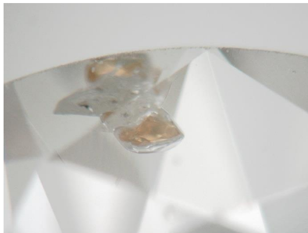
Figure 39. Inclusion de grenat orange écolitique, grossissement x160. Photo © Laboratoire Français de Gemmologie.
