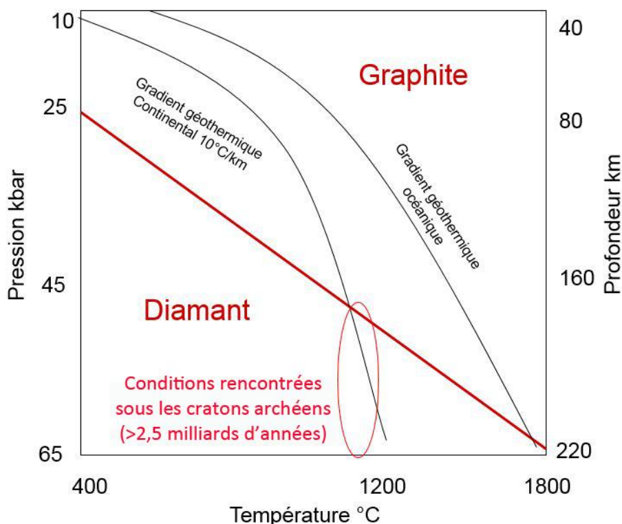
Figure 54. Diagramme de phase du carbone. La zone dans l'ellipse rouge correspond aux conditions terrestres dans lesquelles le diamant peut cristalliser. Ces conditions se retrouvent généralement sous les cratons archéens.
