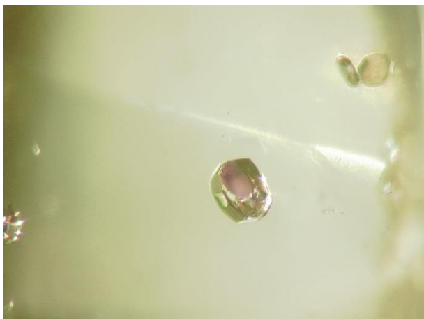
Figure 38. Inclusion cubo-octaédrique d'un pyrope. Le pyrope est un grenat de composition Mg_3Al_2(SiO_4)_3 . Il fait partie de la composition de la péridotite qui est une roche constitutive du manteau supérieur. L'étude des inclusions minérales permettent d'étudier l'origine géologique et la formation des diamants. Photo E. Fritsch.
