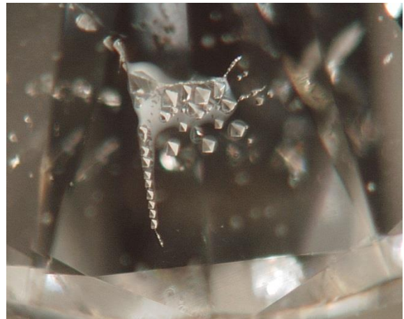
Figure 43. Nuage d'octaèdres négatifs, grossissement x80. Les cristaux négatifs sont des lacunes de cristallisation de la forme du cristal hôte. Photo © Laboratoire Français de Gemmologie.
