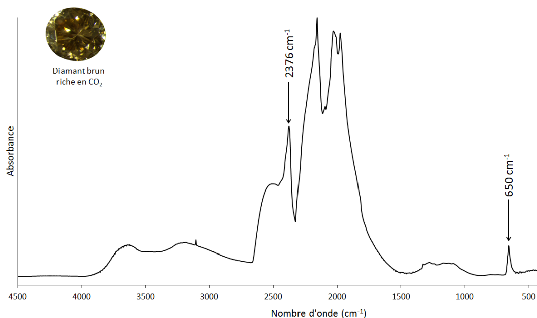
Figure 112. Spectre infrarouge d'un diamant brun à "CO 2 solide". Les absorptions liées au CO 2 sont situées entre 644-660 cm -1 et 2337-2411 cm -1 .
