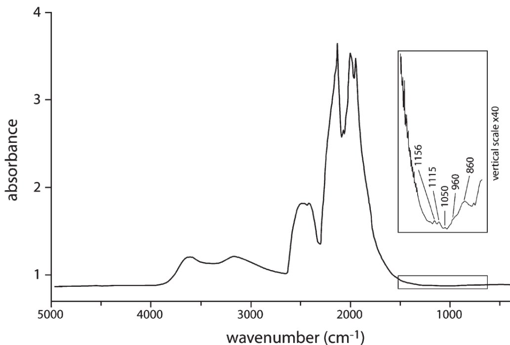
Figure 7. Spectre d'absorption infrarouge du Grand Condé, caractéristique des diamants de type IIa par l'absence d'absorptions majeures dans la zone 500 - 1500 \text{ cm}^{-1} . De petites absorptions non répertoriées dans les diamants de type IIa sont présentes ( 860, 960, 1050, 1115 et 1156 \text{ cm}^{-1} ). Spectre Fritsch et al. (2007).
