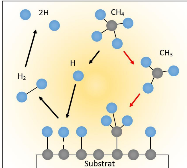
Figure 106. Schéma simplifié du processus de synthèse du diamant CVD. Le plasma permet de casser les molécules. Les hydrogènes présents dans le plasma peuvent ainsi se lier aux hydrogènes de la surface du substrat afin de laisser une liaison carbone pendante. Ainsi la molécule \text{CH}_3 qui a une liaison pendante va pouvoir se lier au substrat par une liaison C-C. Le diamant CVD croît donc en couches.
