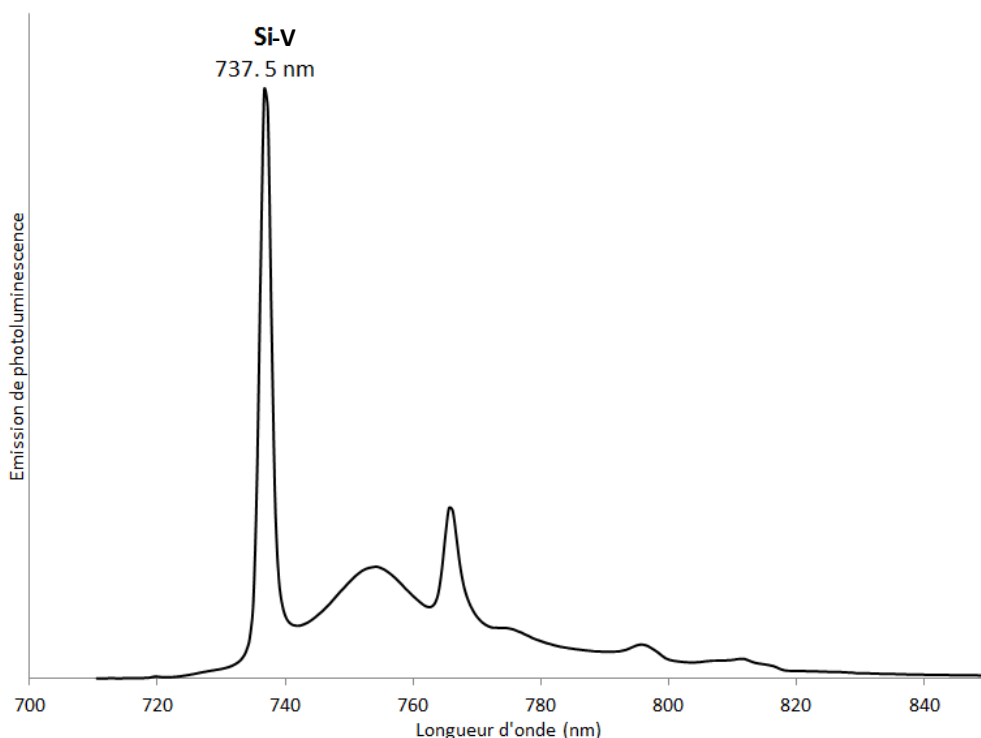
Figure 110. Centre du silicium dans un diamant synthétique CVD à 737,5 nm. Ce centre peut se trouver dans quelques rares diamants naturels.
