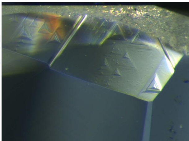
Figure 48. Structures de croissance naturelle du diamant observée sur un naturel, facette brute (non polie) d'un diamant facetté. Photo F.Notari.
