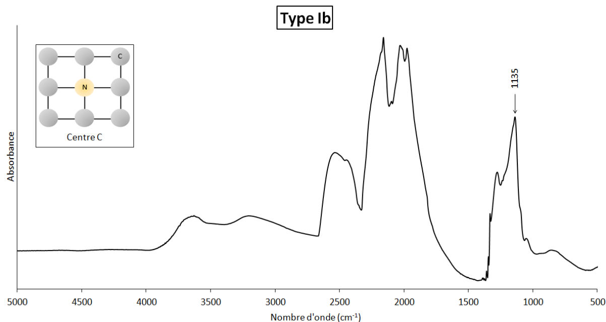
Figure 82. Spectre infrarouge d'un diamant brun de type Ib. La présence d'azote isolé (ou centre C) se traduit par une absorption principale à environ 1135\text{ cm}^{-1} . Ces diamants sont en principe de couleur jaune.
