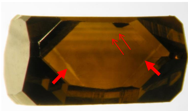
Figure 100. Trace d'un germe à la surface d'un diamant synthétique HPHT. Photo E. Fritsch.
