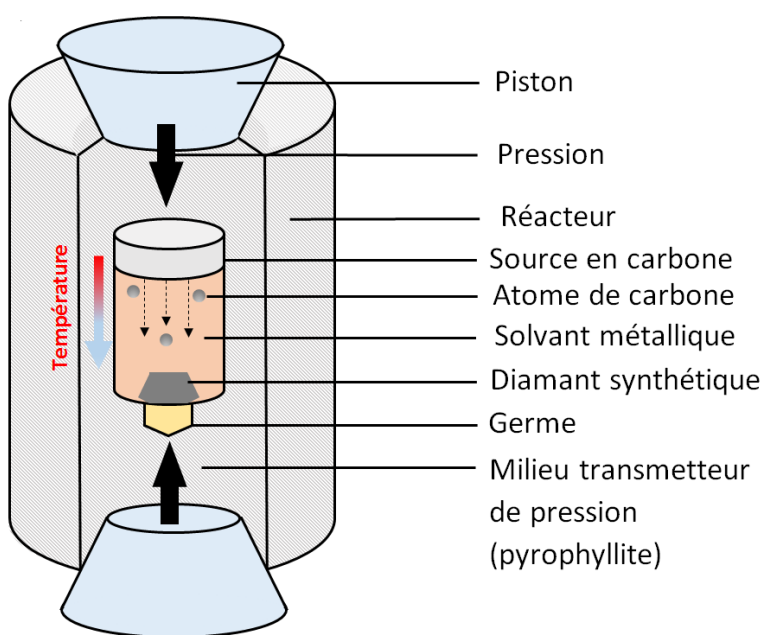
Figure 92. Schéma simplifié d'une presse pour la synthèse du diamant HPHT de type "Belt". Deux pistons, un en haut et un en bas vont faire augmenter la pression à l'intérieur de manière uniaxiale. Un cylindre chauffant (non représenté) à l'intérieur du réacteur va créer un gradient de température dans la cellule haute pression. Ainsi la température sera plus élevée au niveau de la source de carbone et plus "froide" au niveau du germe. Cela permet alors de faire croître un diamant synthétique monocristallin en continuité du germe de diamant dans le solvant métallique.
