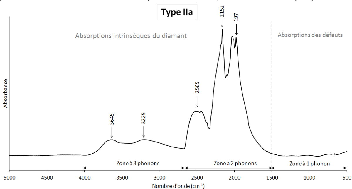
Figure 77. Spectre infrarouge d'un diamant incolore de type IIa. Le spectre est divisé en 3 zones. La zone à 1 phonon ( 400 - 1500 \text{ cm}^{-1} ) est la zone d'absorption des défauts du diamant. Dans le cas du type IIa elle ne présente pas d'absorption. Les zones à 2 et 3 phonons montrent les absorptions intrinsèques du diamant, donc les vibrations des liaisons C-C, les principales étant à 1975 , 2152 , 2505 , 3225 et 3645 \text{ cm}^{-1} . D'après Moutier (2007), modifié.
