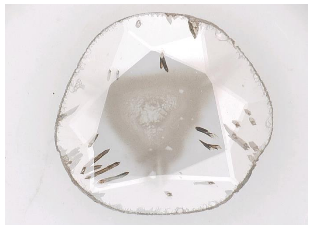
Figure 47. Canaux de Rose dans un diamant, à l'intersection de deux lamelles de macles (Schoor, 2014). Photo E. Fritsch.
