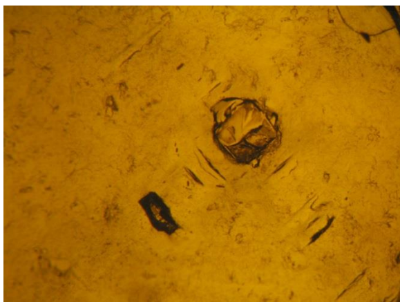
Figure 100. Trace d'un germe à la surface d'un diamant synthétique HPHT. Photo E. Fritsch.
