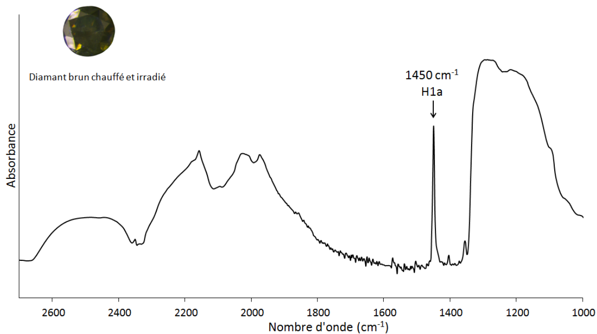
Figure 21. Spectre infrarouge d'un diamant brun irradié et chauffé. Le défaut H1a, à 1450\text{ cm}^{-1} , correspond à une liaison entre un carbone et un azote en position interstitielle.
