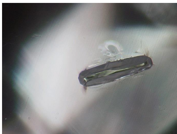
Figure 41. Inclusion de pyroxène dans un diamant, grossissement x150. Le pyroxène communément présent dans les roches du manteau est le diopside CaMg(SiO_3)_2 et se retrouve en inclusion dans le diamant. Photo © Laboratoire Français de Gemmologie.
