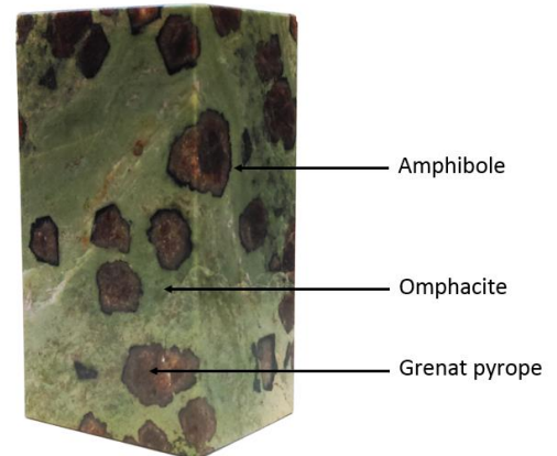
Figure 53. L'éclogite est une roche métamorphique se formant lors d'une subduction. Elle fait partie du manteau et est composée principalement d'omphacite (pyroxène), de grenat pyrope et d'amphibole qui se forme entre l'omphacite et le grenat.
