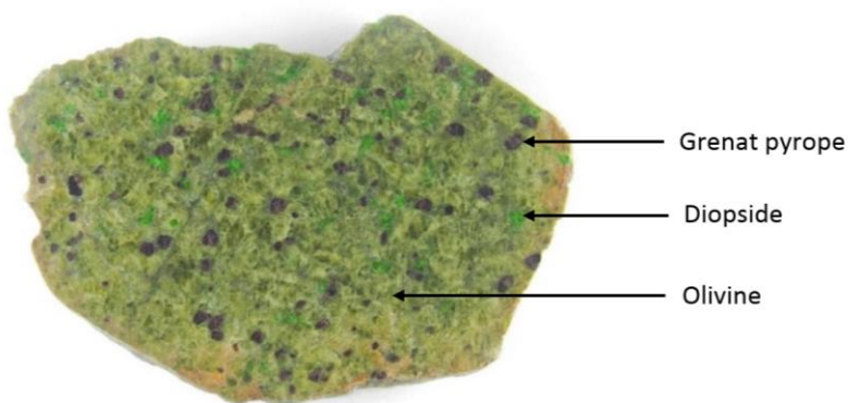
Figure 52. La péridotite est la roche constitutive majeure du manteau supérieur terrestre. Elle se compose d'olivine, de diopside chromifère (pyroxène) et de grenat pyrope. Des morceaux de cette roche sont souvent arrachés lors de la remontée du magma et forme les xénolites dans les kimberlites. Photo B.Rondeau.
