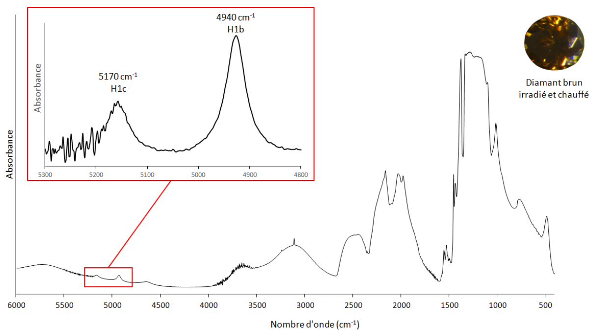
Figure 22. Spectre infrarouge d'un diamant irradié et chauffé. H1b ( 4940\text{ cm}^{-1} ) et H1c ( 5170\text{ cm}^{-1} ) apparaissent après irradiation et chauffage des diamants de type Ia.
