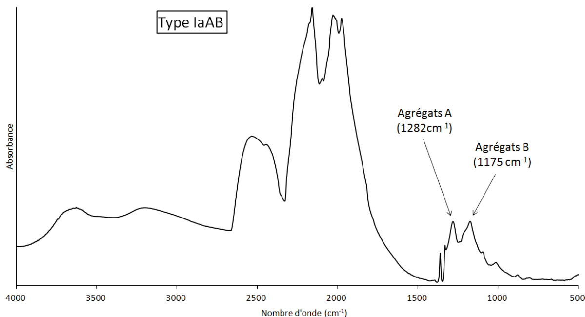
Figure 81. Spectre infrarouge d'un diamant brun de type IaAB avec une absorptions des agrégats A environ égale à celle des agrégats B. Les diamants de type IaAB présentent les absorptions dans la zone à 1 phonon des deux agrégats, 1175\text{ cm}^{-1} pour les agrégats B et 1282\text{ cm}^{-1} pour les agrégats A.
