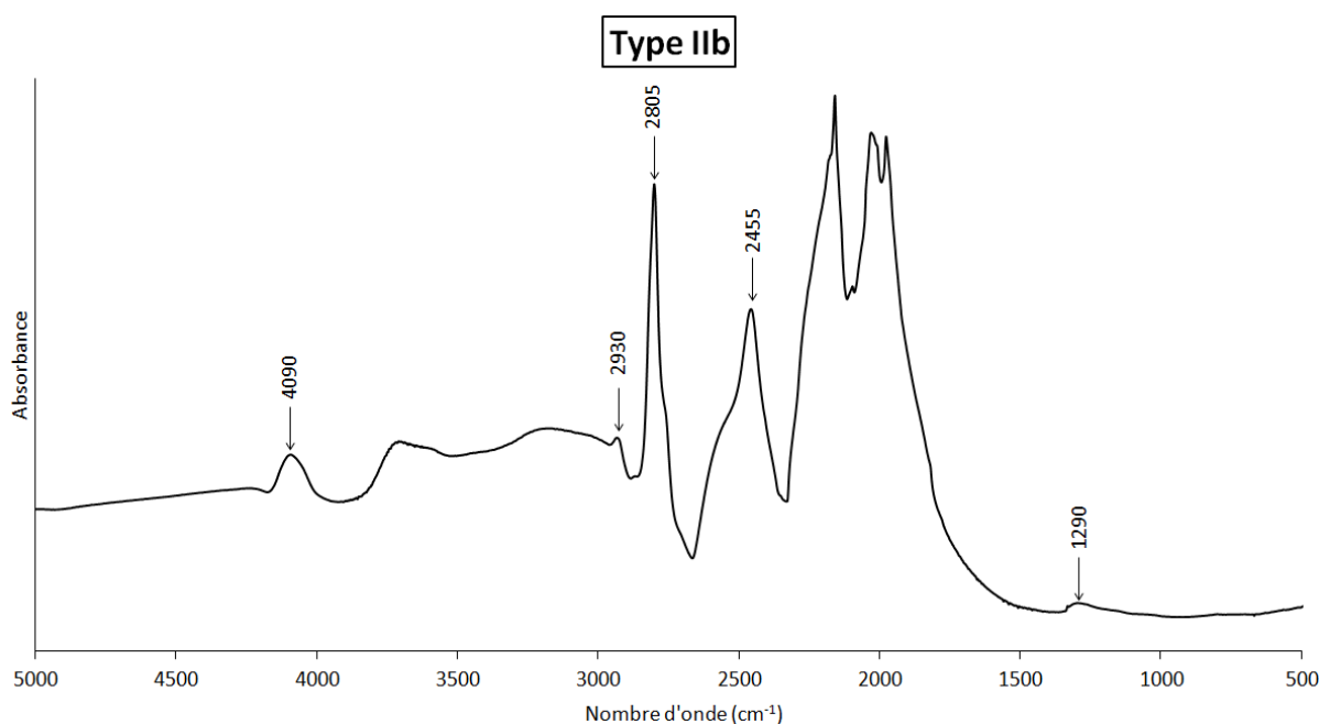
Figure 78. Spectre d'absorption d'un diamant de type IIb. Les diamants de type IIb peuvent être de couleur bleue ou grise. Le spectre, en plus de présenter les absorptions intrinsèques du diamant, comporte des absorptions liées au bore qui absorbe dans les zones à 1, 2 et 3 phonons aux nombres d'onde suivant : 1290, 2455, 2805, 2930 et 4090 \text{cm}^{-1} .
