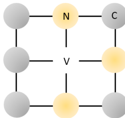
Figure 23. Schéma simplifié en 2D du centre N3. Ce centre est composé de 3 atomes d'azotes entourant une lacune.
