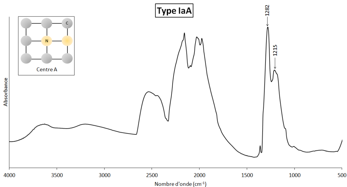
Figure 79. Spectre infrarouge d'un diamant de type IaA. Les diamants de type IaA présentent deux absorptions principales liées aux agrégats A à 1282\text{ cm}^{-1} et 1215\text{ cm}^{-1} dans la zone à 1 phonon.
