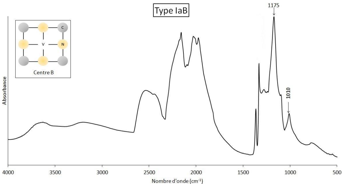
Figure 80. Spectre infrarouge d'un diamant de type IaB. Les diamants de type IaB présentent deux absorptions dans la zone à 1 phonon lié aux agrégats B ( 1175 et 1010\text{ cm}^{-1} ).
