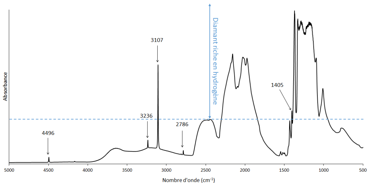
Figure 26. Spectre infrarouge d'un diamant riche en hydrogène. Les pics engendrés par les liaisons C-H se situent principalement à 1405, 2786, 3107, 3236 et 4496 \text{cm}^{-1} . De plus ce diamant est considéré comme "riche en hydrogène" puisque l'absorbance du pic à 3107 \text{cm}^{-1} est supérieure à l'absorbance de la bande à 2450 \text{cm}^{-1} .
