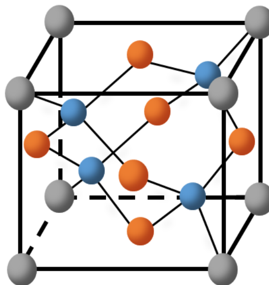
Figure 8. Schéma de la maille cristalline du diamant. Le diamant cristallise dans le système cubique composé de 8 atomes de carbone aux sommets du cube (gris), 6 atomes au centre des faces (orange) et 4 en site Td (bleu).
