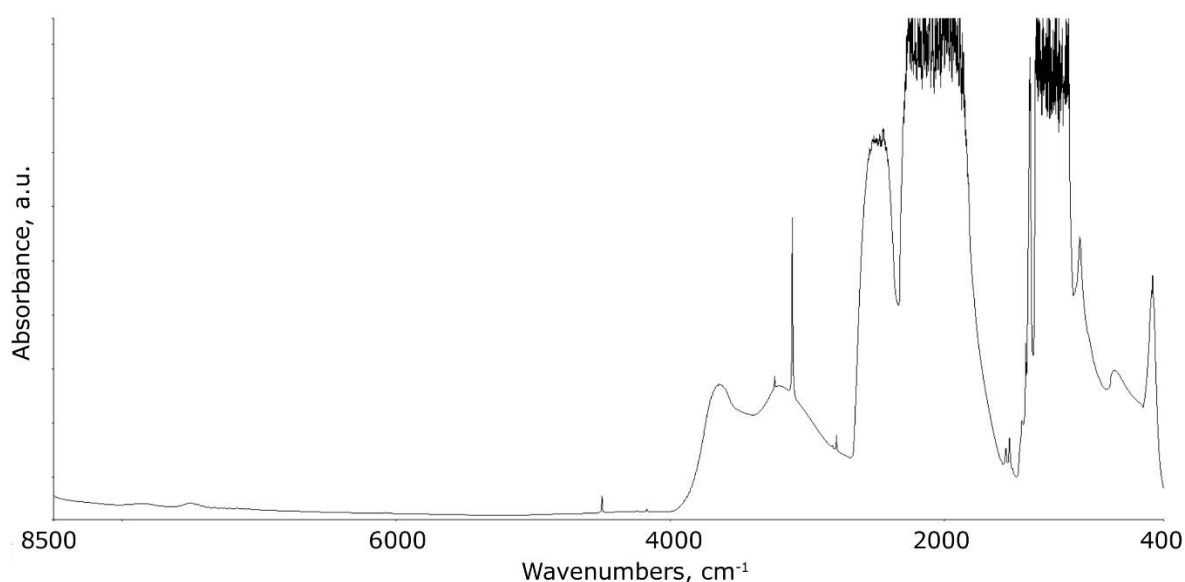
Figure 4. Spectre infrarouge de l'Œil du Tigre, diamant brun de type IaA>B riche en azote et en hydrogène (pic à 3107\text{ cm}^{-1} ). Spectre © GGTL Laboratories 2016.
