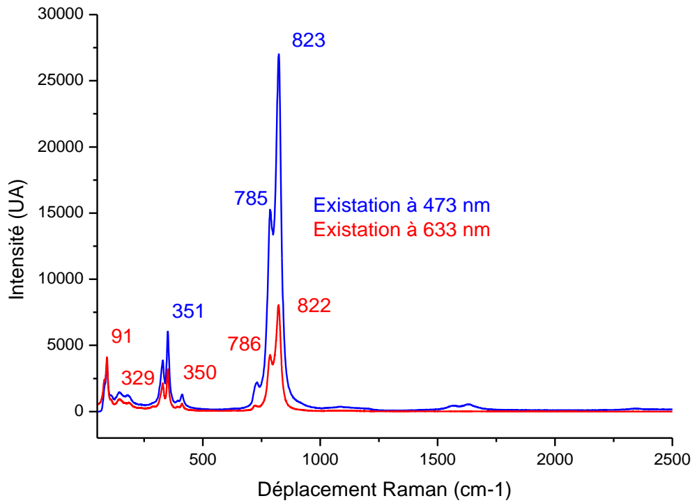
R. vanadinite échantillon 10,23 ct graphique de comparaison à 473 nm et à 633 nm
