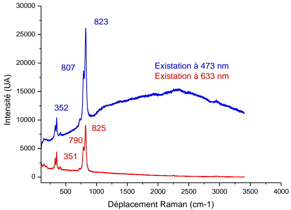
R. vanadinite échantillon 36,40 ct graphique de comparaison à 473 nm et 633 nm
