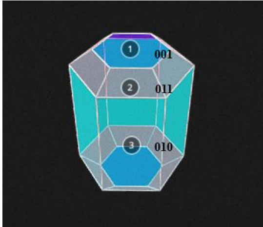
FIGURE 12 : D'APRÈS DES DESSINS DE « L'ATLAS DER KRYSTALLFORMEN » DE VM GOLDSCHMIDT (1913-1923)
