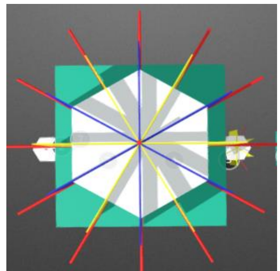
FIGURE 11,10 : HTTPS://SKETCHFAB.COM/3D-MODELS/HEXAGONAL/ VUE DE FACE ET VUE DE HAUT TOUTS LES ÉLÉMENTS DE SYMÉTRIE
