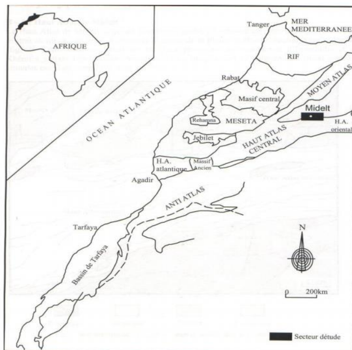
FIGURE 3 : LES DIFFÉRENTS DOMAINES STRUCTURAUX DU MAROC ET LOCALISATION DU SECTEUR D'ÉTUDE (IGMOULLAN ET AL. 1987)
