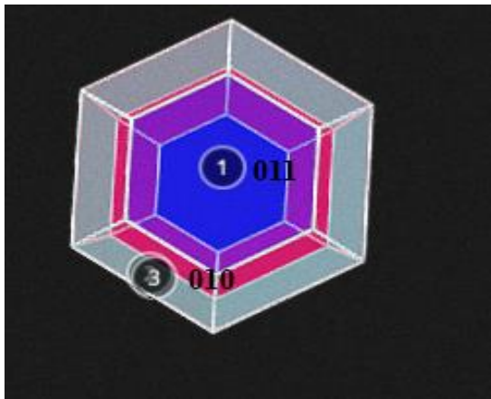
FIGURE 13 : FACE DU DESSUS / D'APRÈS DES DESSINS DE « L'ATLAS DER KRYSTALLFORMEN » DE VM GOLDSCHMIDT (1913-1923)
