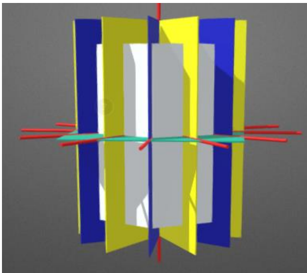
FIGURE 11,10 : HTTPS://SKETCHFAB.COM/3D-MODELS/HEXAGONAL/ VUE DE FACE ET VUE DE HAUT TOUTS LES ÉLÉMENTS DE SYMÉTRIE
